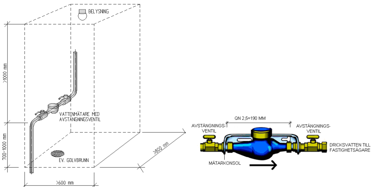
Figur 1 Vattenmätarplatsens utseende och utrymmesbehov.
